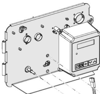
Moteur CC
